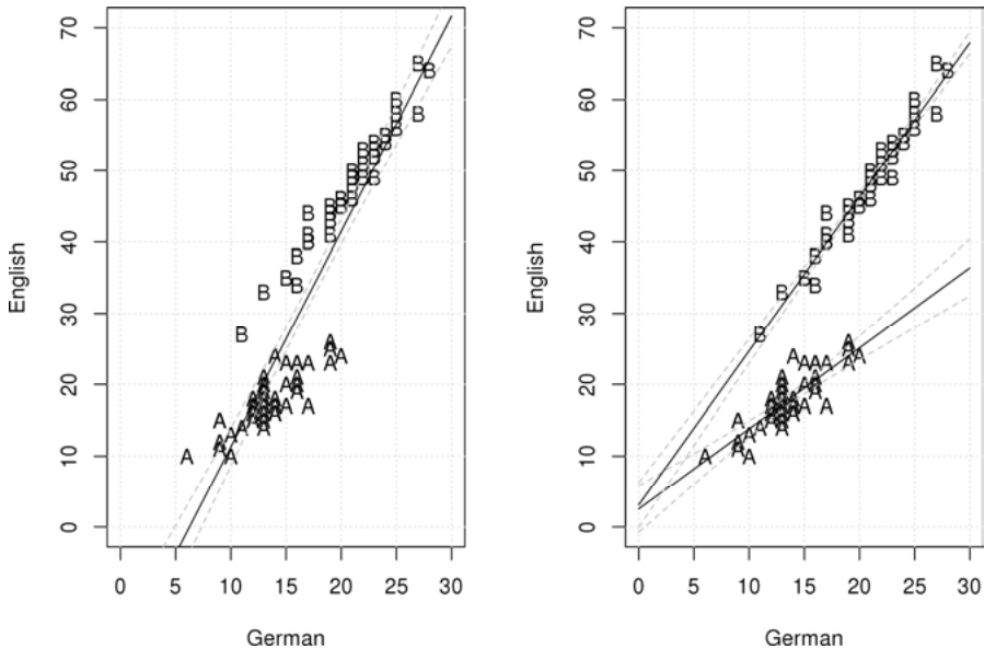
Figure 61. \text{ENGLISH} \sim \text{GERMAN} + \text{CLASS} (+ \text{GERMAN}:\text{CLASS})
